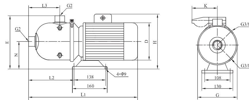
安装图
