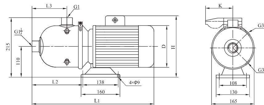
安装图
