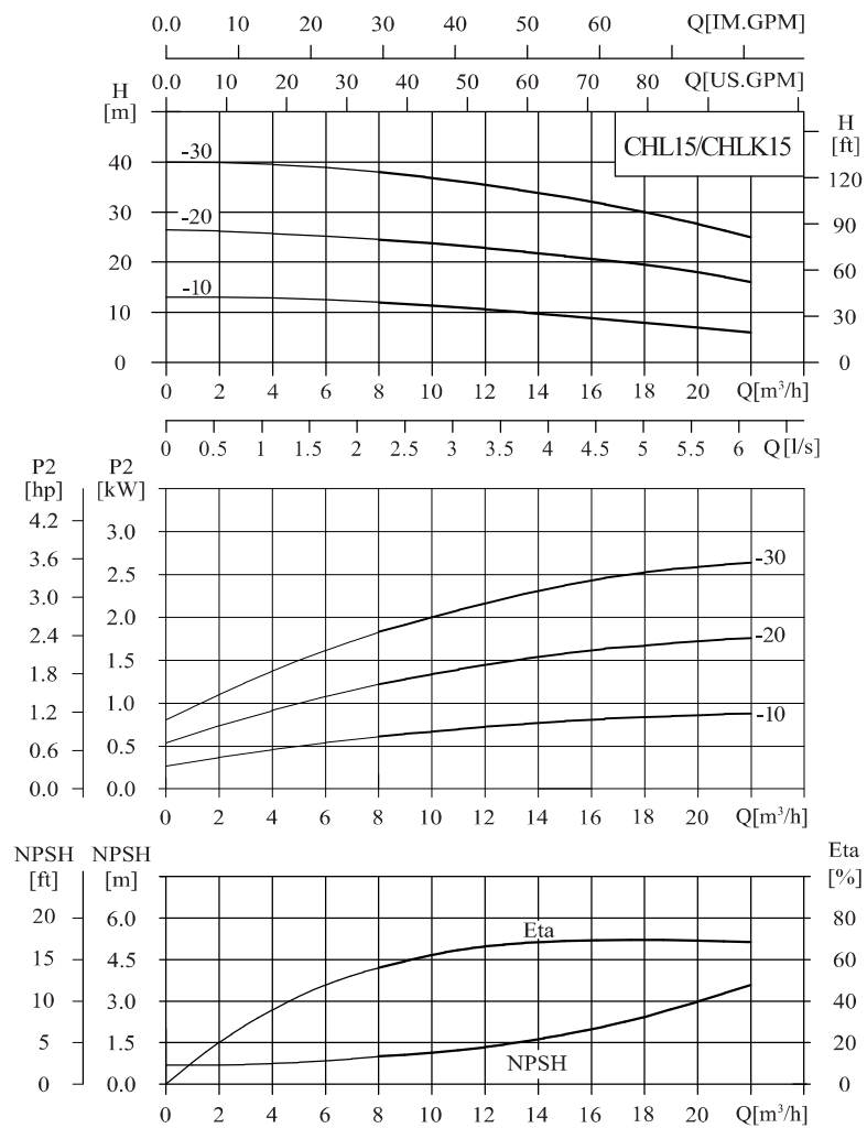
性能曲线
