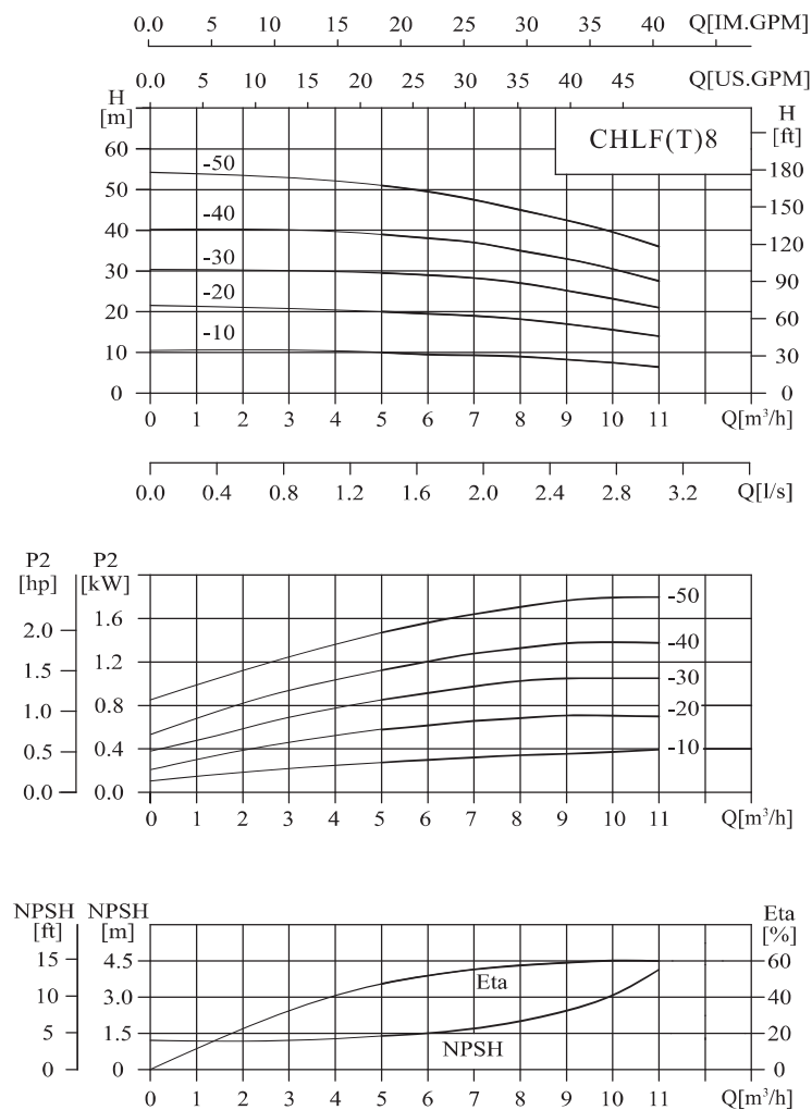
性能曲线
