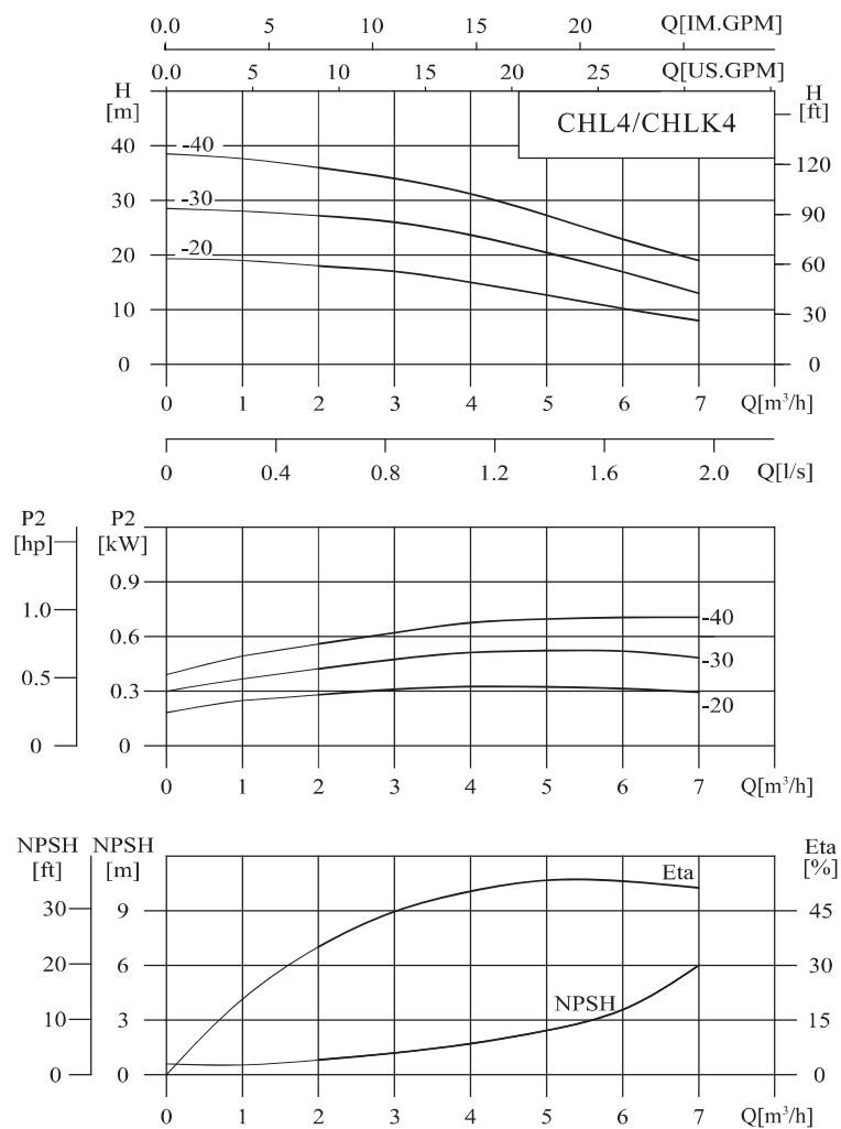
性能曲线
