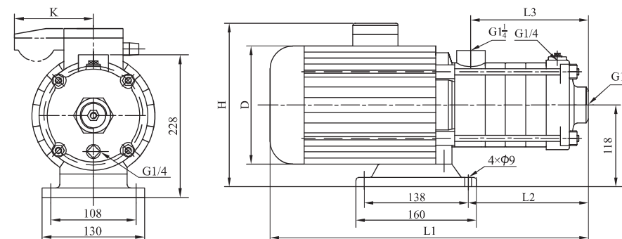
尺寸和重量
